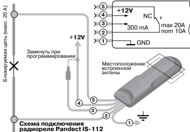
Схема подключения радиореле Pandect IS-112
